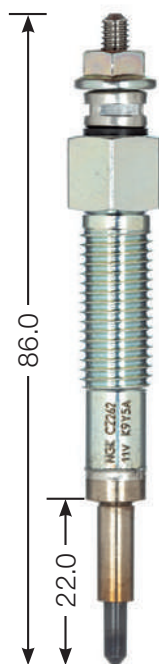
CZ 262 M 10 x 1.25 12 Hex 11 V DP 13
