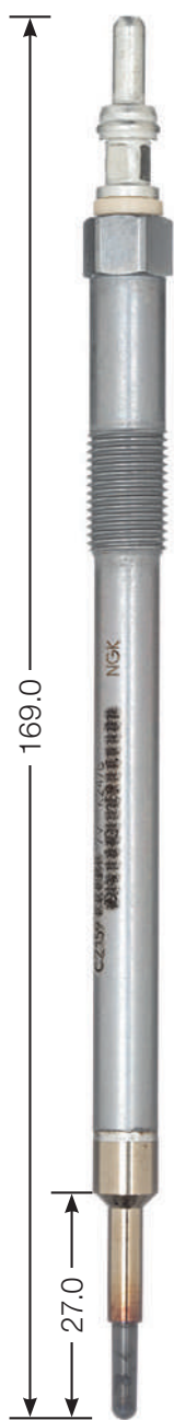
CZ 159 M 10 x 1.0 10 Hex 7 V DP 84
