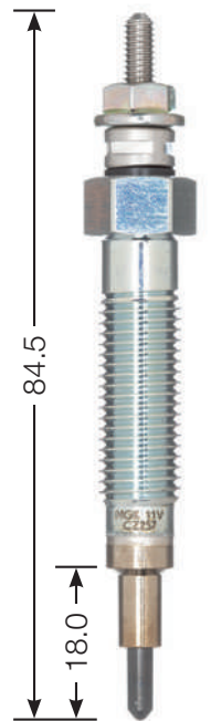
CZ 257 M 10 x 1.25 12 Hex 11 V DP 83
