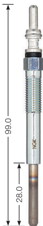
YE 08 M 8 x 1.0 8 Hex 11 V
