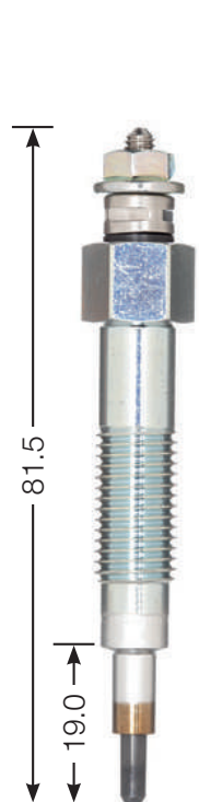
CZ 259 M 10 x 1.25 12 Hex 11 V
